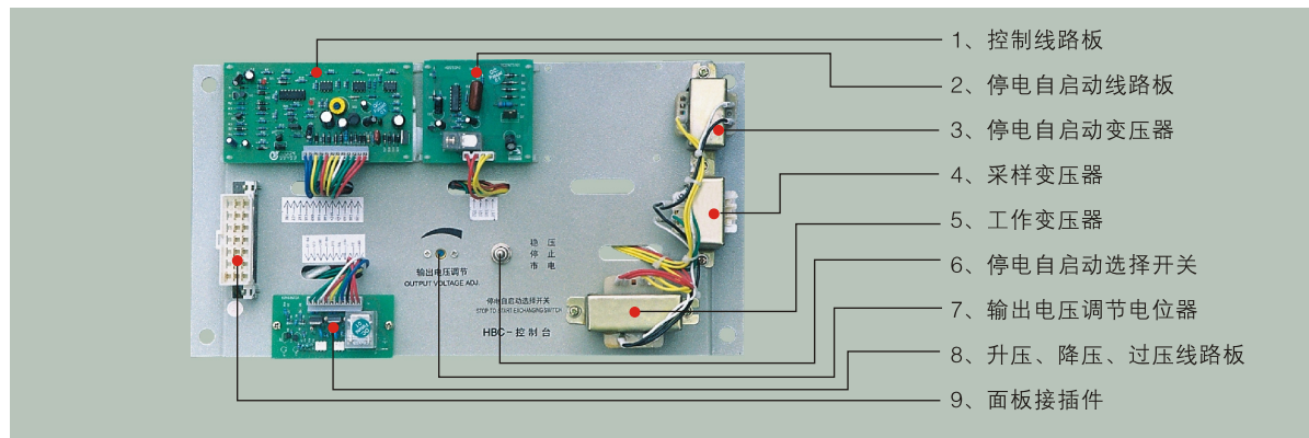
20-60KVA 控制台
