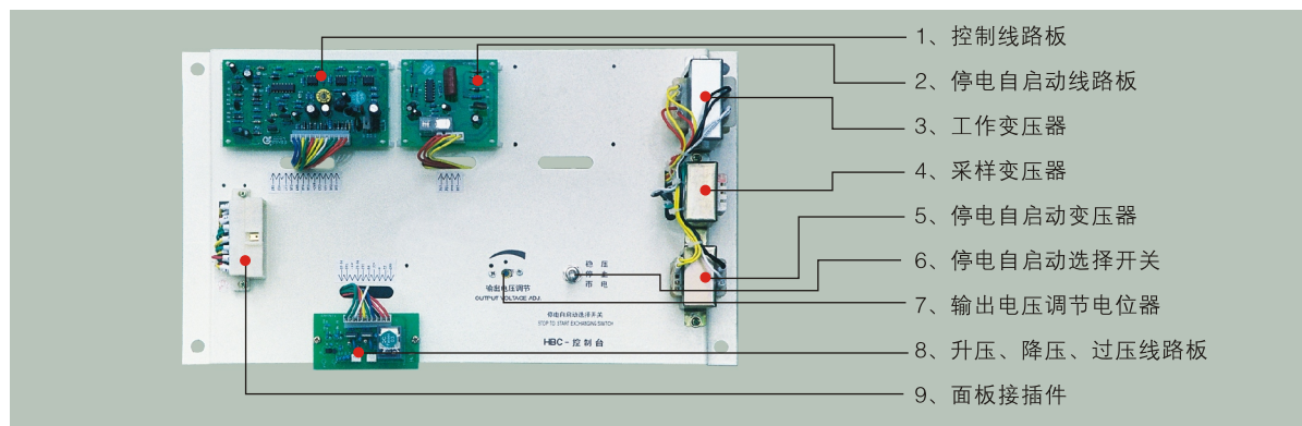
80-120KVA 控制台
